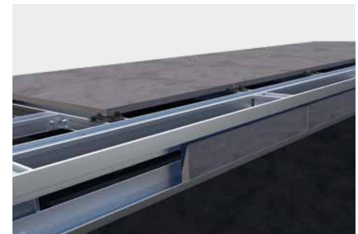
Anwendungsbeispiel Abschlussprofile Alu-Unterkonstruktion
