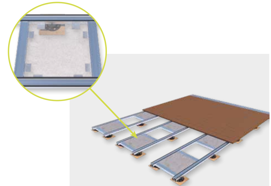
Windsogsicherung bei Holzterrassen mit Betonplatten und Auflastwinkel.
