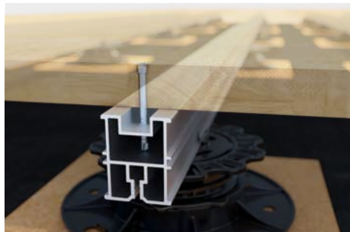
Anwendungsbeispiel Alu-Systemprofil TERRA H50
