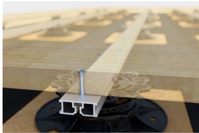
Anwendungsbeispiel Alu-Systemprofil TERRA H15
