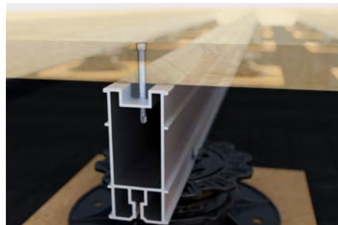
Anwendungsbeispiel Alu-Systemprofil TERRA H85
