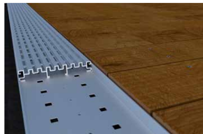
DrainTec Base in Kombination mit dem DrainTec Drainagerost ohne Unterkonstruktion.
