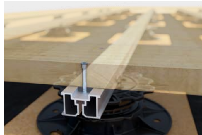
Anwendungsbeispiel Alu-Systemprofil TERRA H24
